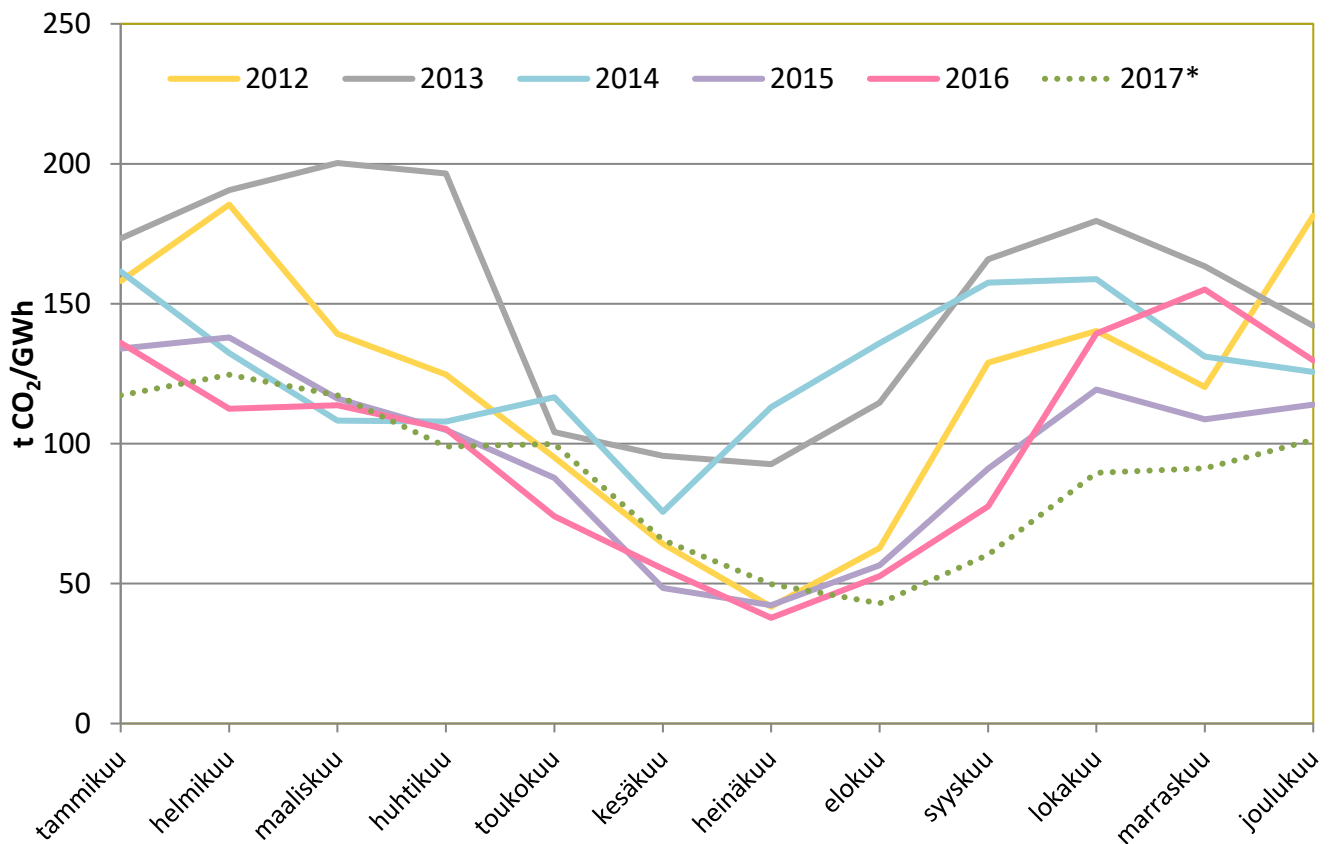
Kuva 1. Sähkönkulutuksen päästökerroin kuukausitasolla vuosina 2012–2017, laskettuna hyödynjakomenetelmällä Energiategollisuus ry:n aineistosta. Vuoden 2017 tieto on ennakkotieto.
