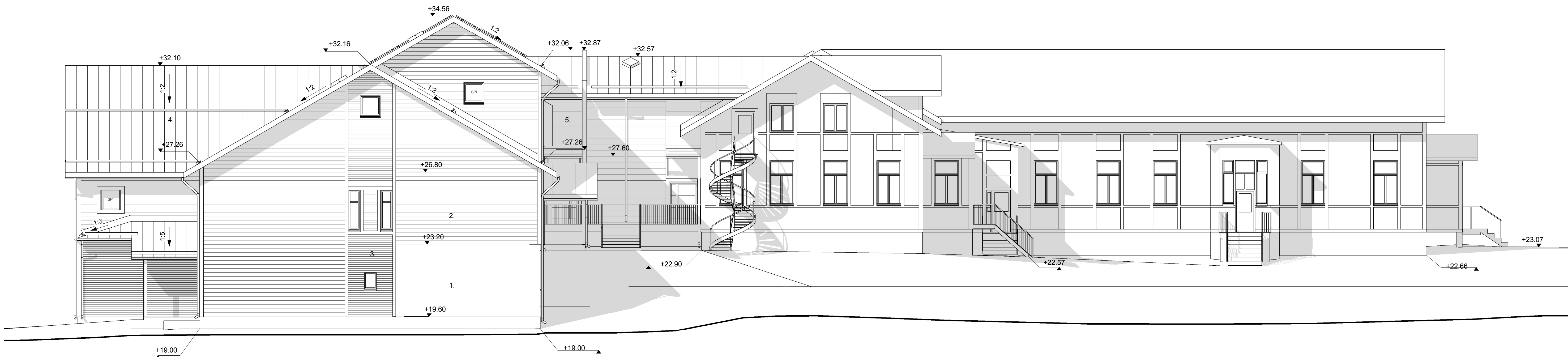
JULKISIVU POHJOISEEN
