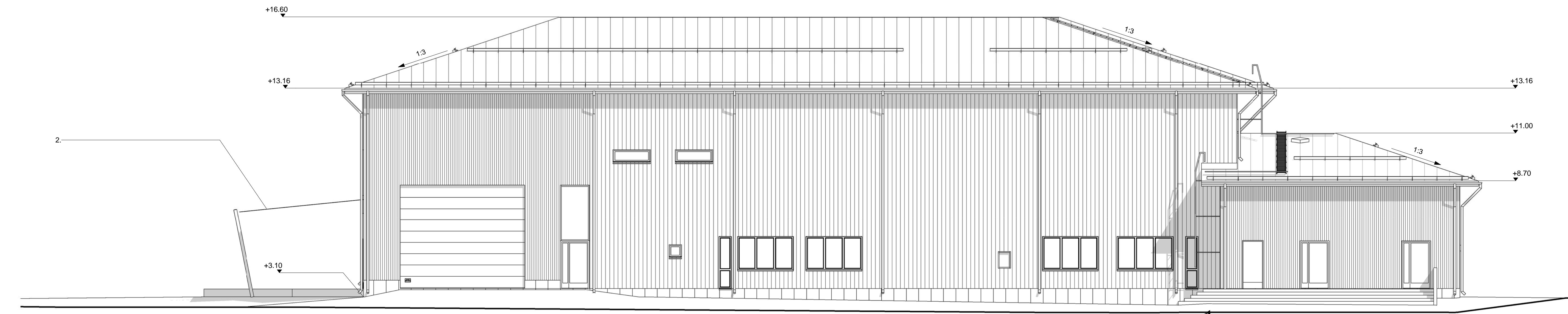
LUOTEeseen 1 : 100
