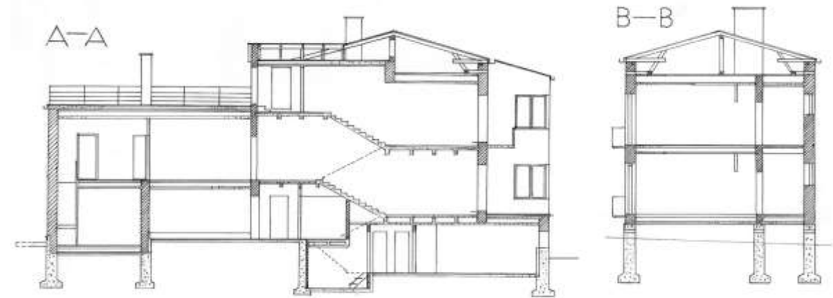
Kuva 7. Leikkaukset A-A ja B-B, joista ensimmäisissä näkyy siipien välinen korkeusero ja yhteys "huoltosiiven" kattoterassille. B-B leikkaus on huoneistosiivestä.
