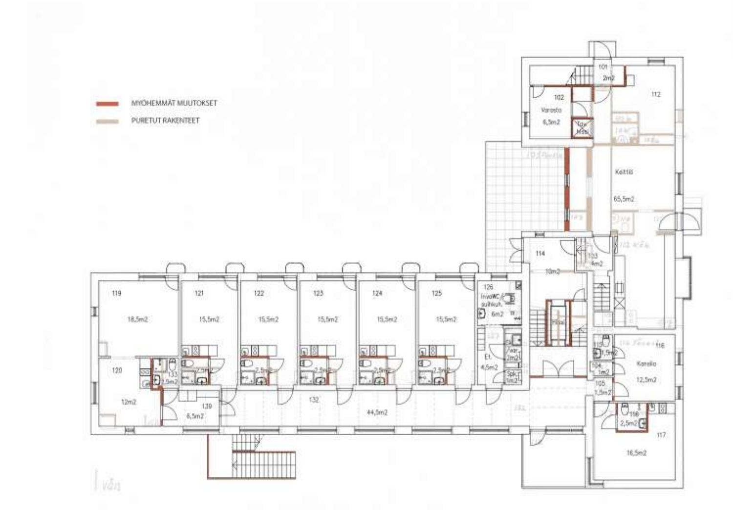
Kuva 16. Ensimmäisen kerroksen pohjapiirros.
