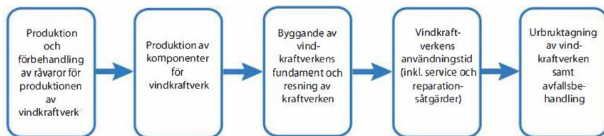
Figur 2-2. Vindkraftverkens livscykel
