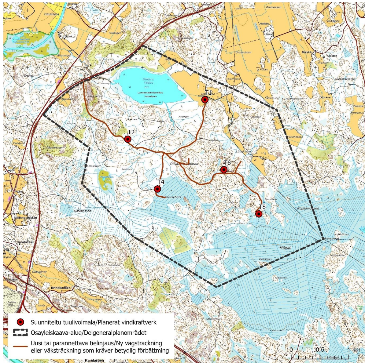
Figur 6-2. Enskilda vägar.
