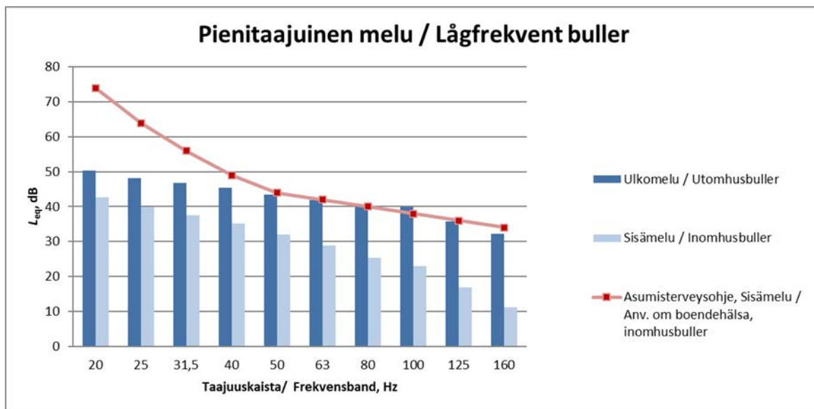
Figur 6-21. Beräkningsresultat för lågfrekvent buller vid jämförelsepunkt 1.
