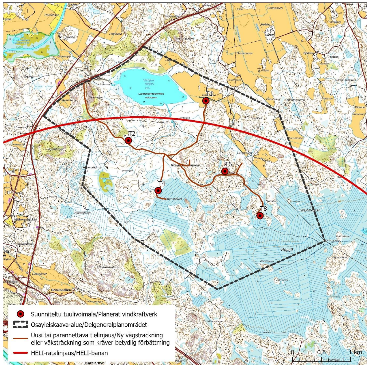
Figur 6-5. Vägförbindelser som ska förbättras och HELI-banans sträckning.
