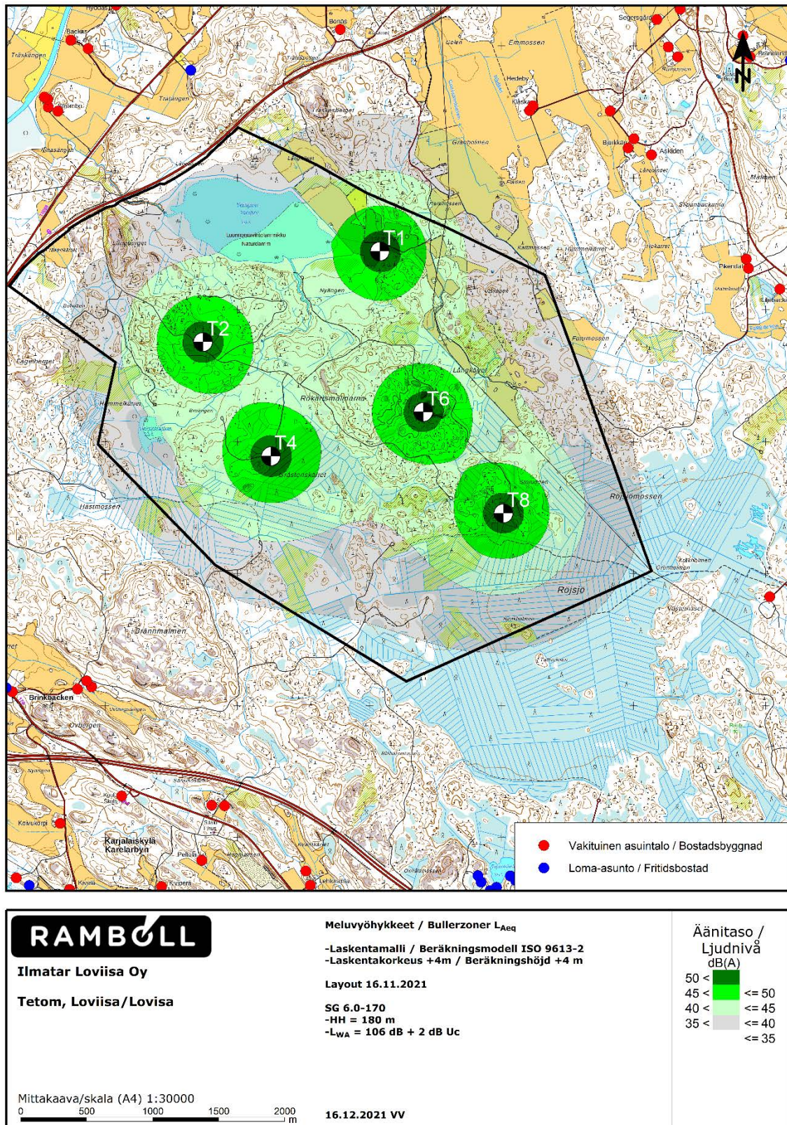
Figur 6-20. Resultat av bullermodelleringen då vindkraftverkens ljudeffektnivå är 108,1 dB.
