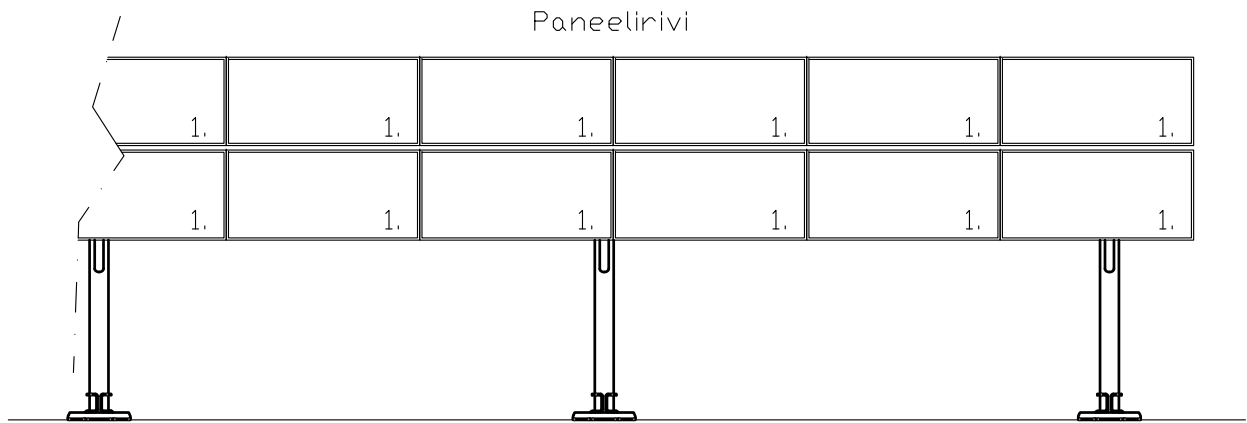
Julkisivu etelään
